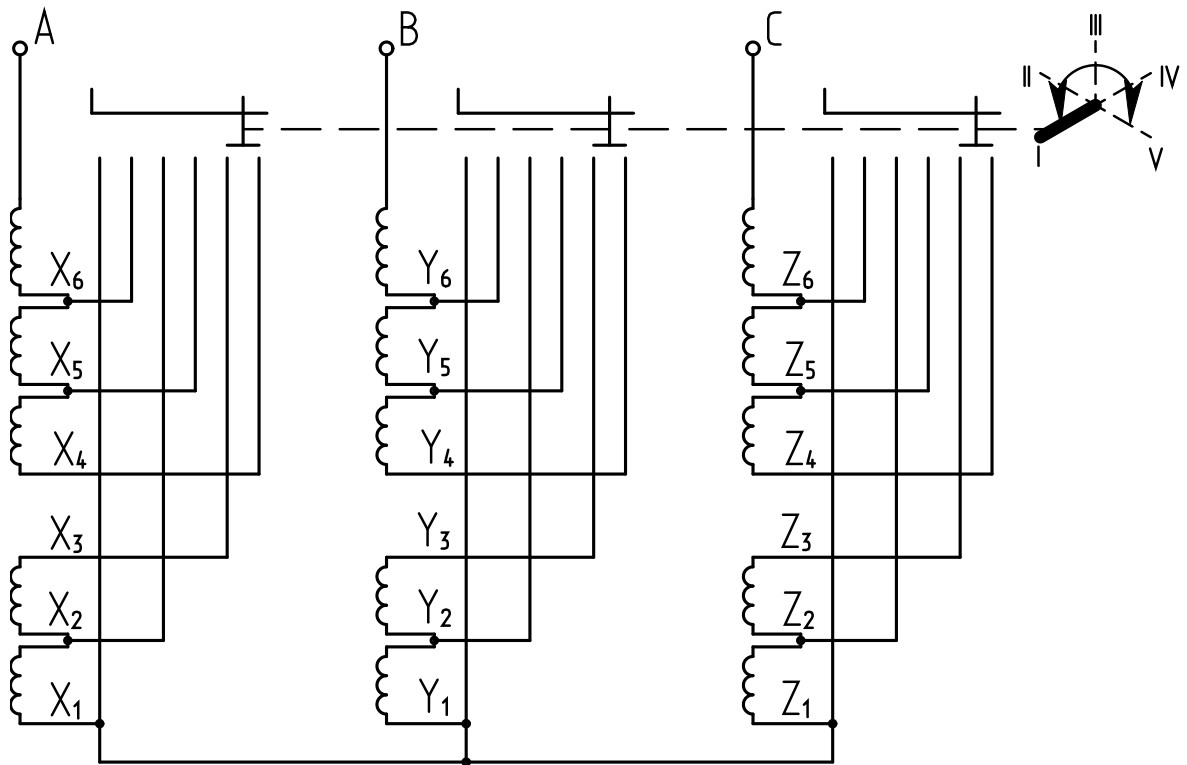
Рисунок А.11 – Схема подключения ответвлений обмоток ВН к переключателю при схеме соединения обмоток – «ЗВЕЗДА»
