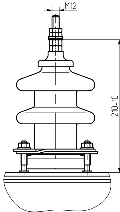
Рисунок А.5 – Вводы ВН
