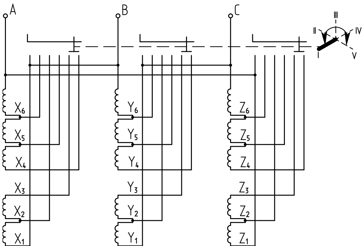
Рисунок А.12 – Схема подключения ответвлений обмоток ВН к переключателю при схеме соединения обмоток – «ТРЕУГОЛЬНИК»
