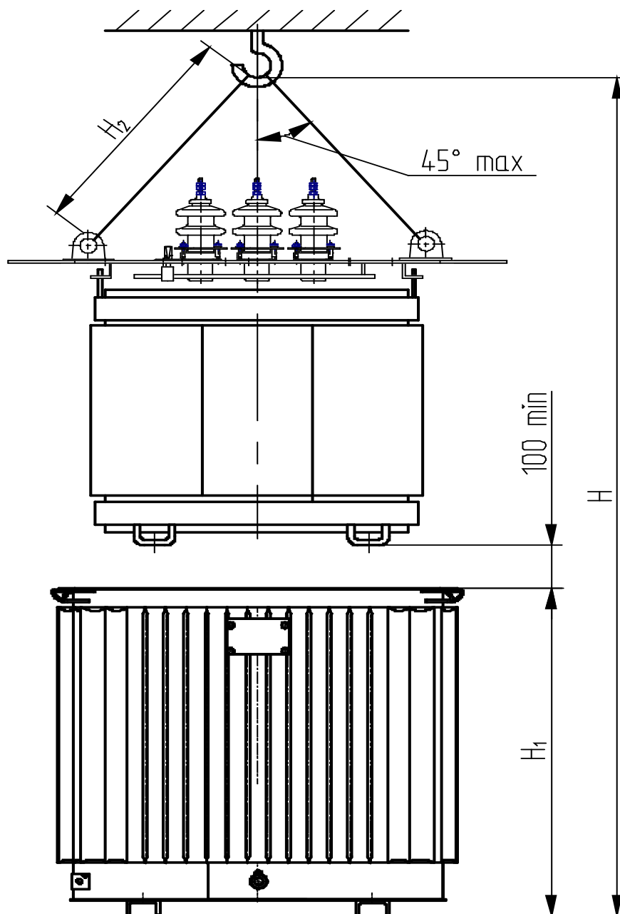
Рисунок А.18 – Эскиз подъема активной части с крышкой
